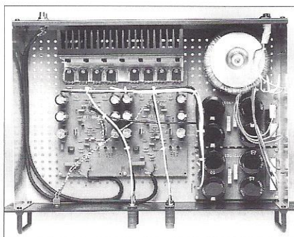
Compleet gemonteerde A-18 versterker
